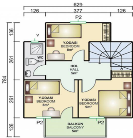
38 m 2 + 5 m 2 = 43 m 2 1.Kat Planı / First Floor Plan
